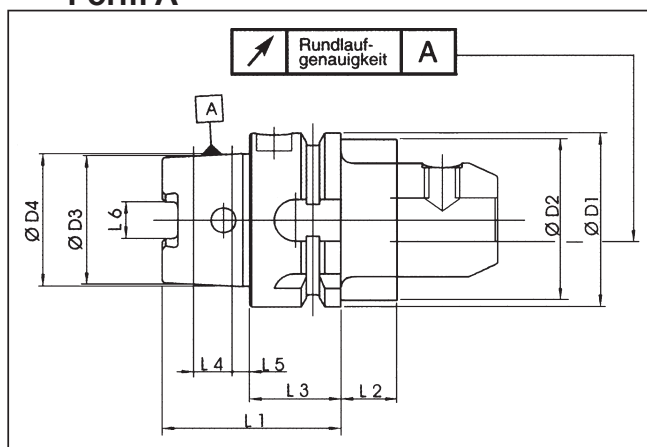
DIN 69893
