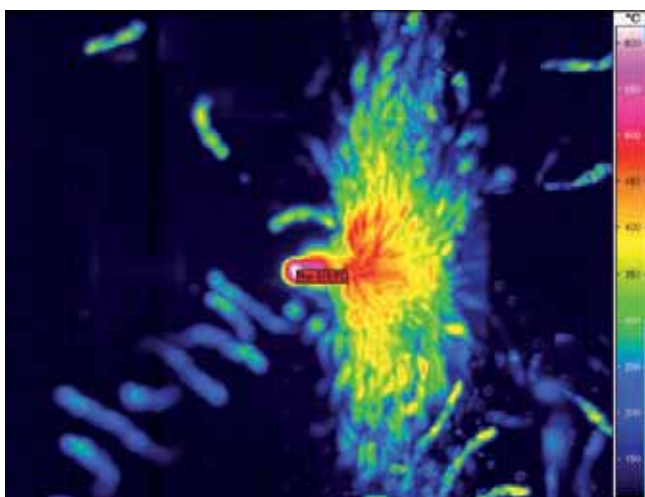
\vartheta_{\max} : 619 °C
