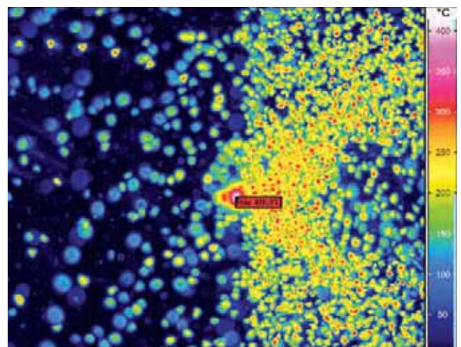
\vartheta_{\max} : 416 °C
